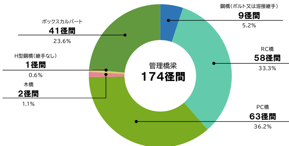
図 4 橋種別の橋梁数(径間数)
