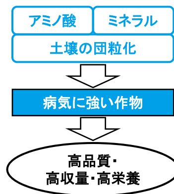
BLOF理論の概略図
